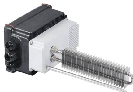
带内置翅片式加热器和空气温度传感器的温度控制器
